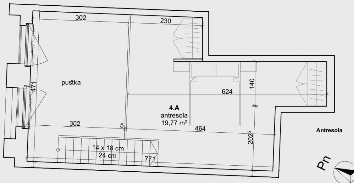
Rzut piętra
